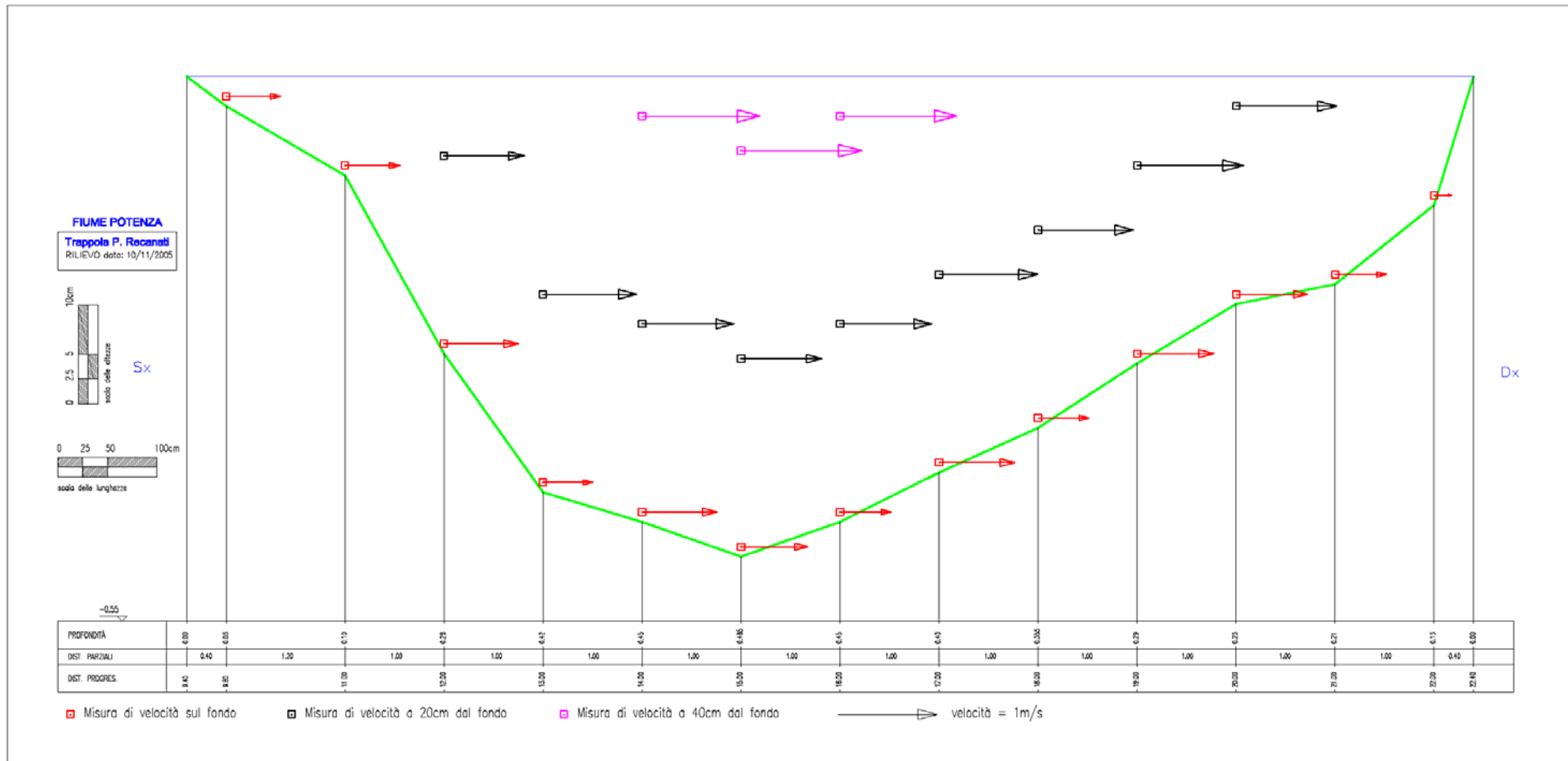
Figura 7.15 - Rilievi idrometrici nella sezione della trappola in località "Foce Potenza"
