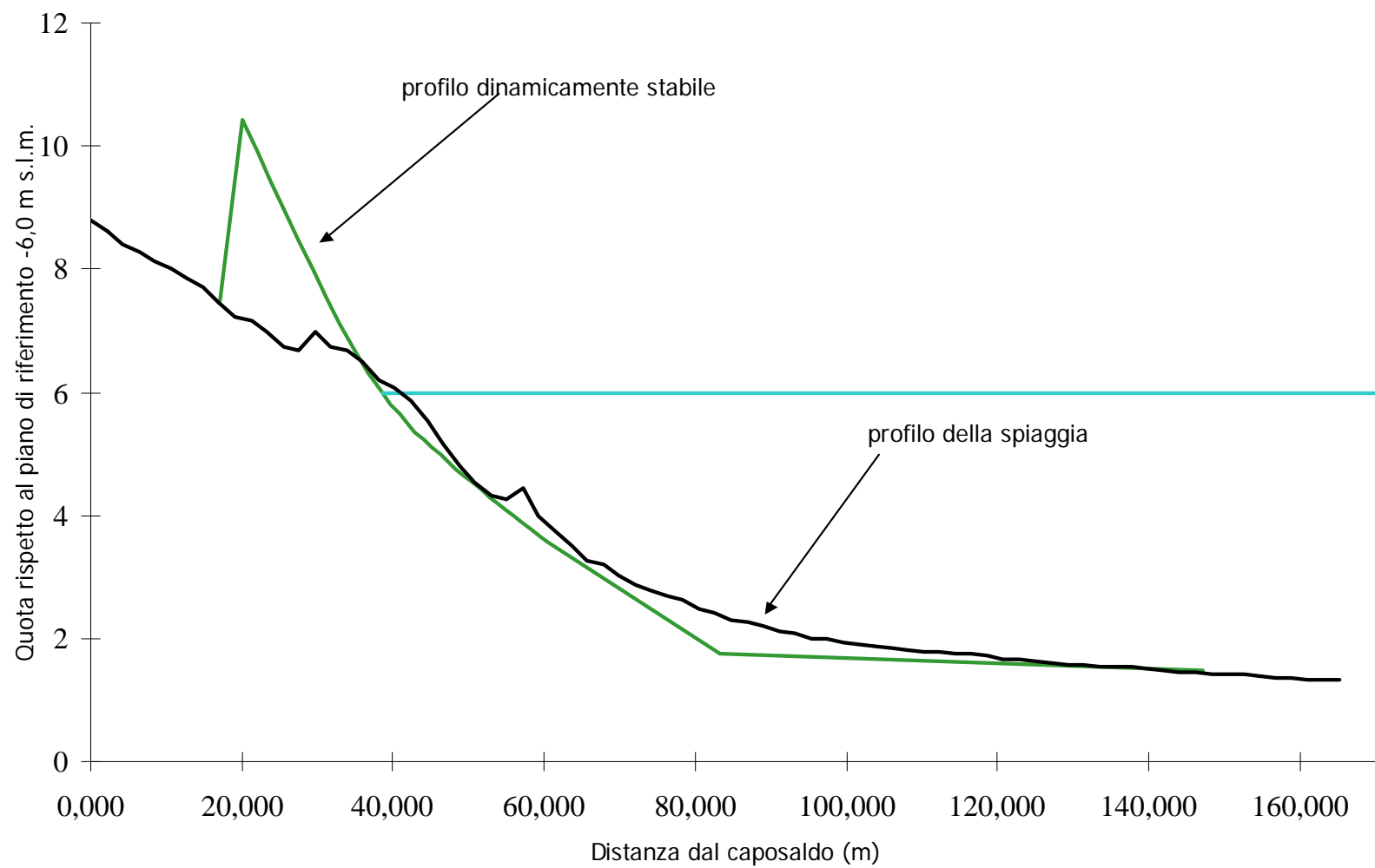
Figura 6.6 - Profilo dinamicamente stabile relativo al profilo iniziale della costa 169-1 e utilizzando i dati ondosi medi.
