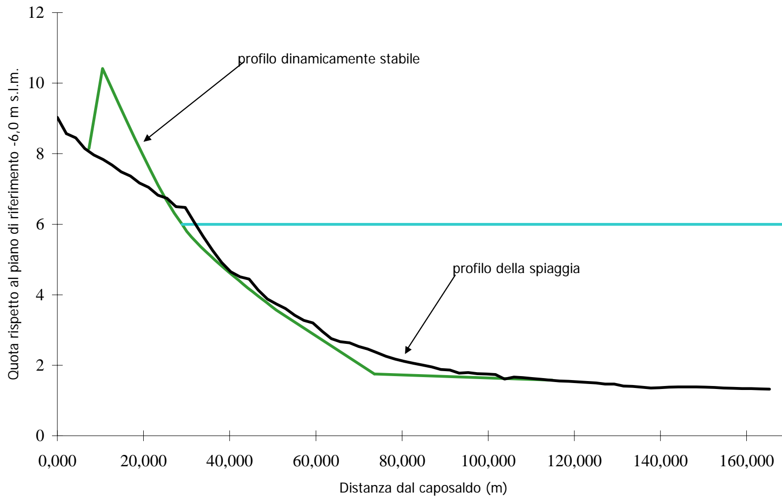
Figura 6.8 - Profilo dinamicamente stabile relativo al profilo iniziale della costa 168-2 e utilizzando i dati ondosi medi.
