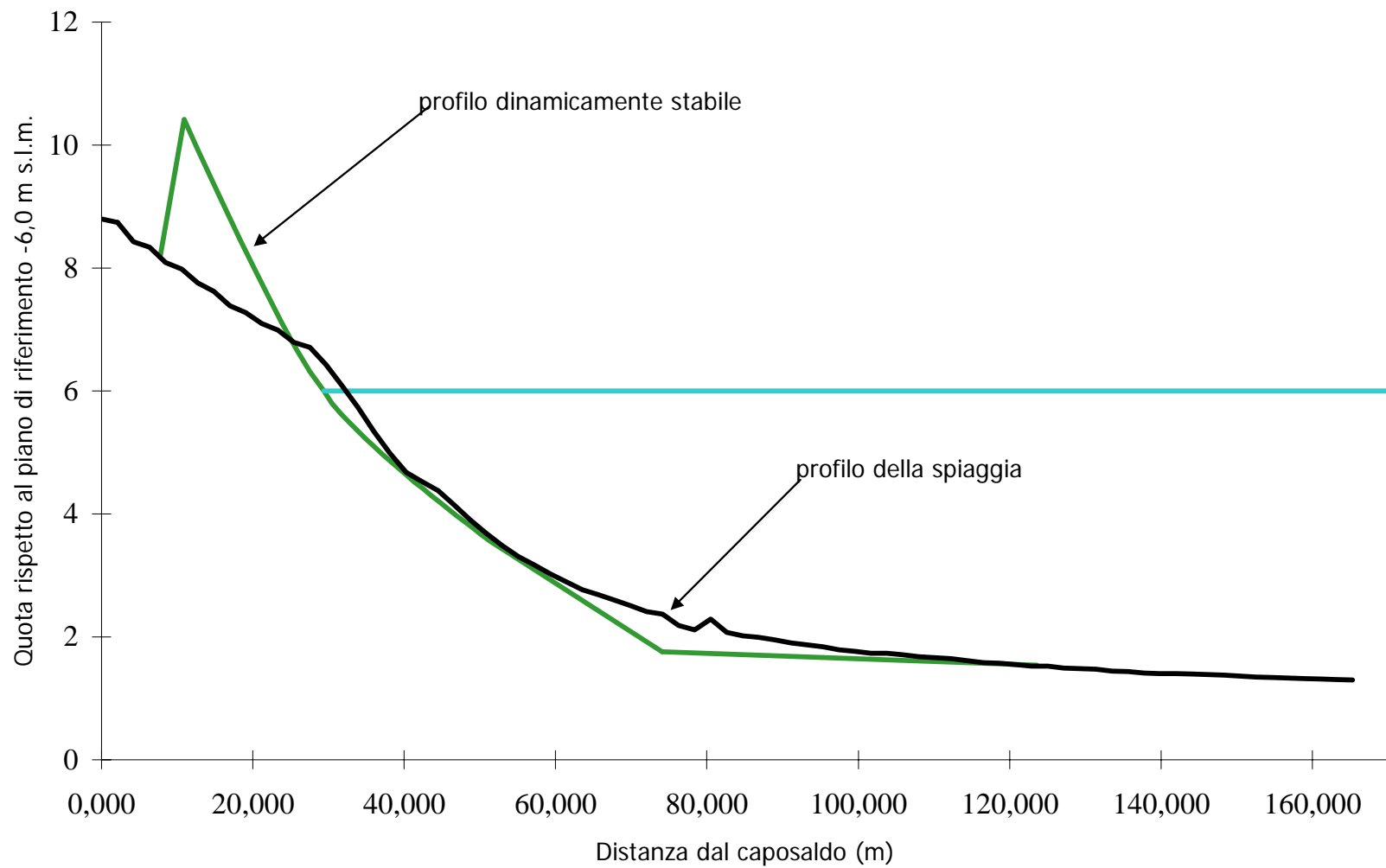
Figura 6.7 - Profilo dinamicamente stabile relativo al profilo iniziale della costa 168-3 e utilizzando i dati ondosi medi.
